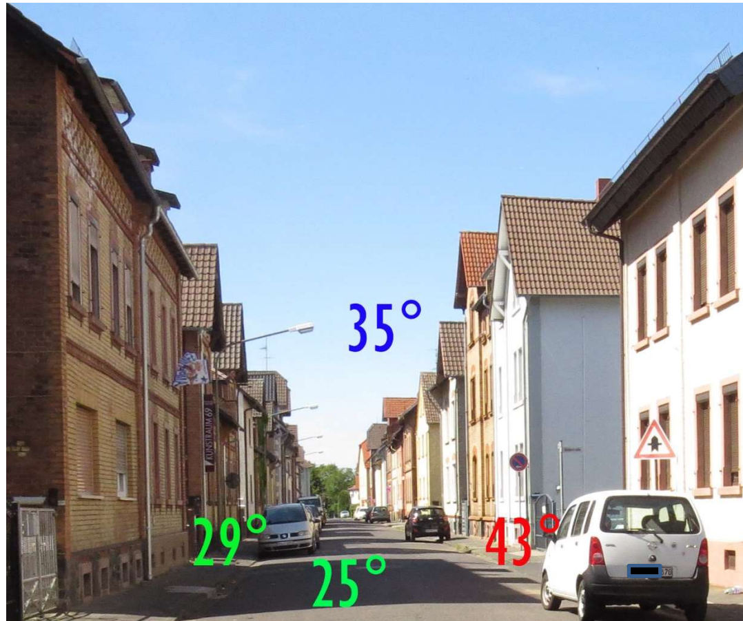
Oberflächentemperaturen Auwanneweg, Großauheim, am 05.08.2018 bei einer Lufttemperatur von 35 °C
